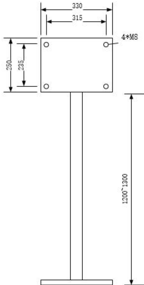
操作柱安装尺寸图
